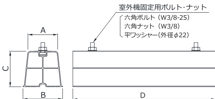
寸法図
