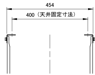
天井固定板内向き取付け
