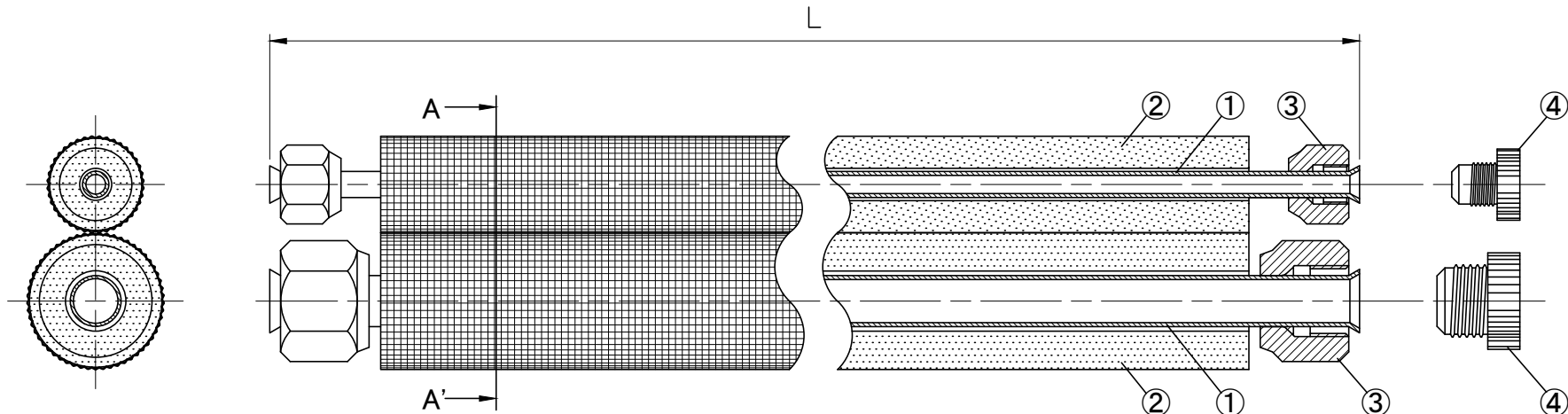
A-A断面
