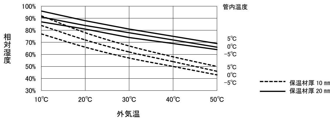
図-9 銅管 \phi 31.75
