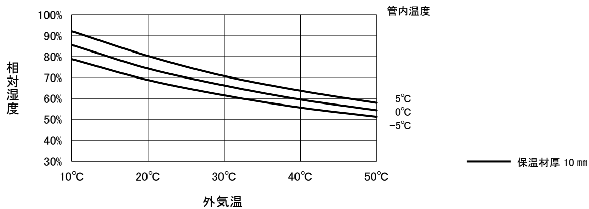
図-11 銅管 \phi 6.35
