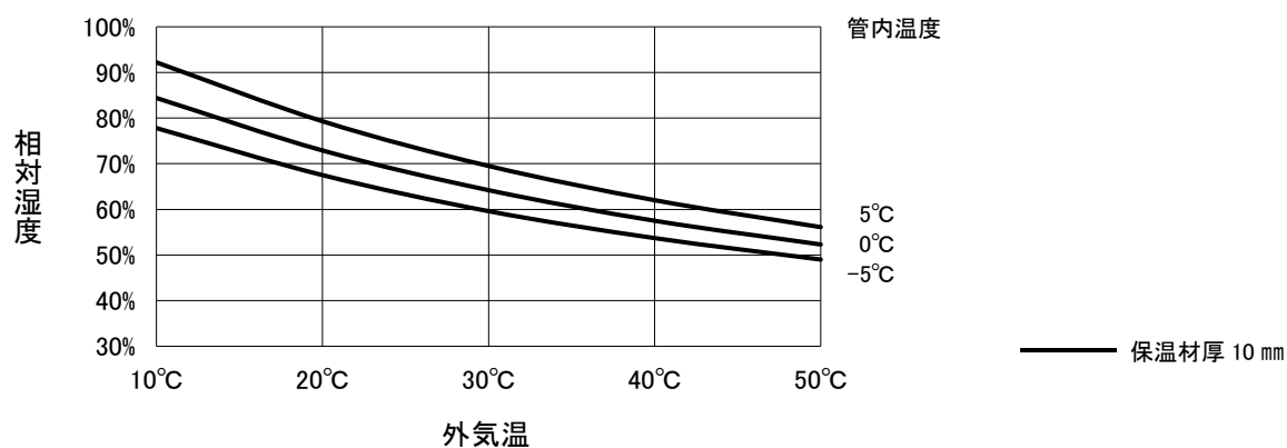
図-12 銅管 \phi 9.52
