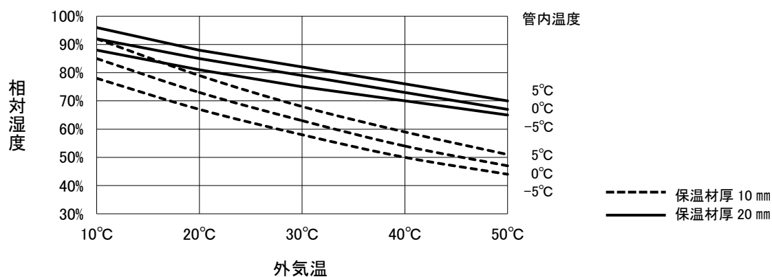
図-7 銅管 \phi 25.40
