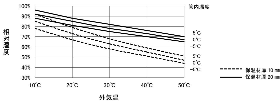
図-8 銅管 \phi 28.58
