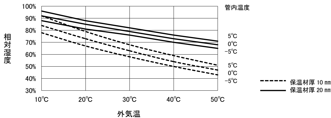
图-6 铜管 \phi 22.22
