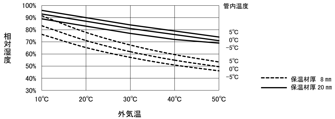
図-4 銅管 \phi 15.88
