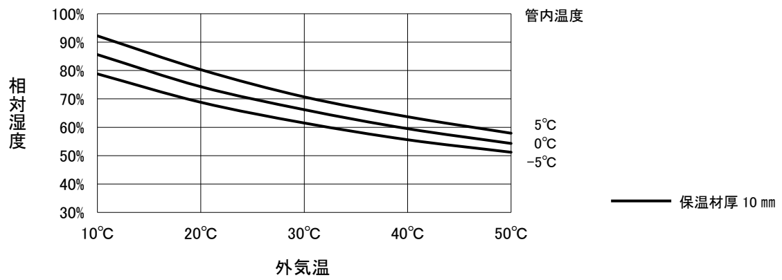
図-5 銅管 \phi 6.35
