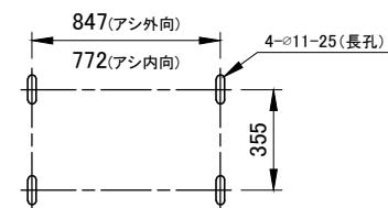
アンカー固定寸法
