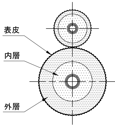
A-A'断面
